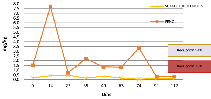
Evolución Temporal FENOL Y CLOROFENOLES. Reactor M5- con Estiércol
