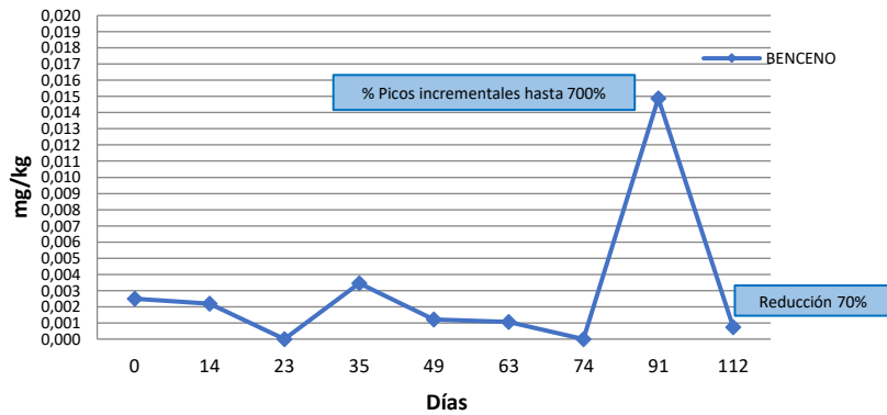
Evolución temporal BENCENO. Reactor AE2- con estiércol
