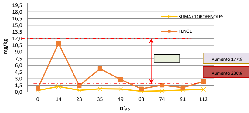
Evolución Temporal FENOL Y CLOROFENOLES. Reactor AN4. Con Estiércol
