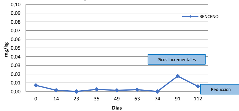
Evolución temporal BENCENO. Reactor AN3. Sin Estiércol
