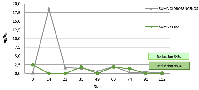
Evolución temporal ETTEX-CLOROBENCENO Reactor AE6- con Estiércol
