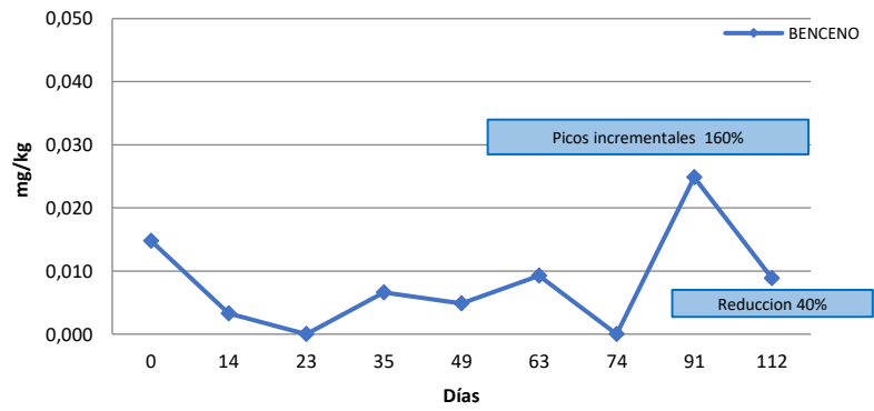
Evolución temporal Benceno -Reactor AE6 Estiércol
