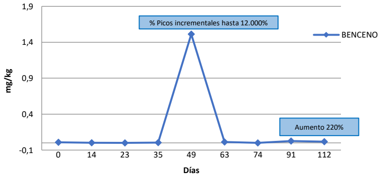
Evolución temporal Benceno. Reactor M5 con Estiércol
