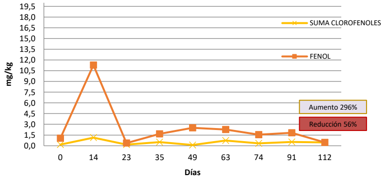
Evolución Temporal FENOL Y CLOROFENOLES. Reactor AN3. Sin Estiércol
