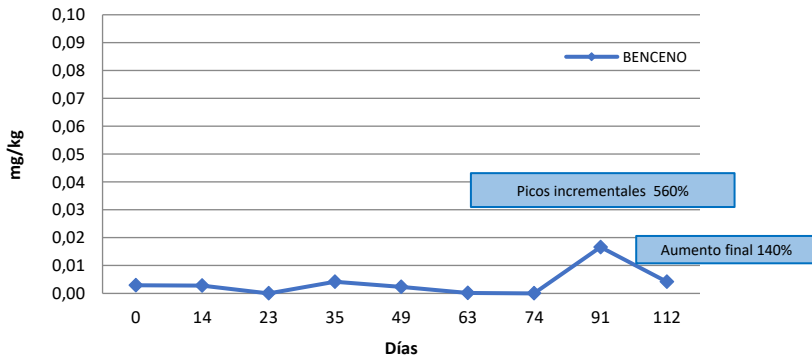
Evolución temporal BENCENO. Reactor AN4. Con Estiércol
