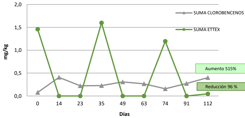
Evolución temporal ETTEX-CLOROBENCENO. Reactor AN3. Sin Estiércol
