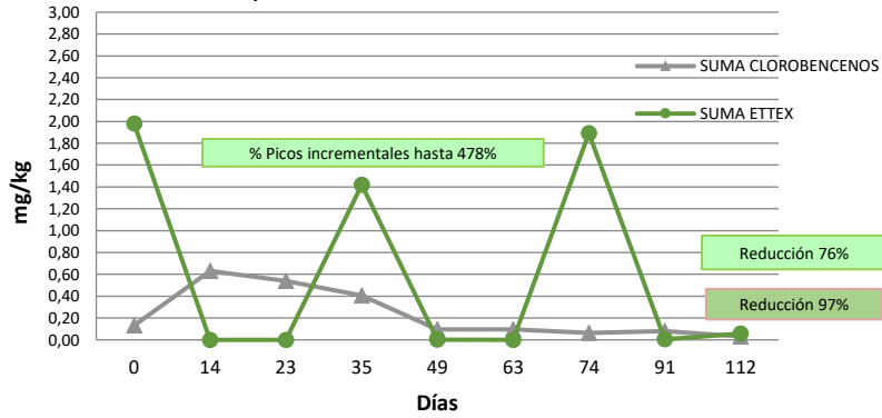
Evolución temporal ETTEX-CLOROBENCENOS. Reactor AE2 - con estiércol
