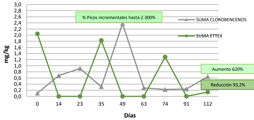
Evolución temporal ETTEX-CLOROBENCENO Reactor M5 - con Estiércol
