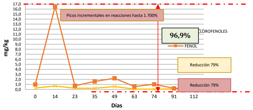
Evolución Temporal FENOL Y CLOROFENOLES. Reactor AE2-con Estiércol
