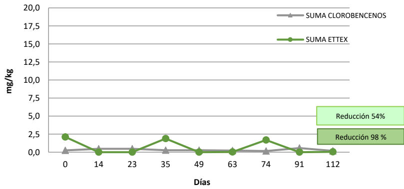
Evolución temporal ETTEX-CLOROBENCENO. Reactor AN4. Con Estiércol
