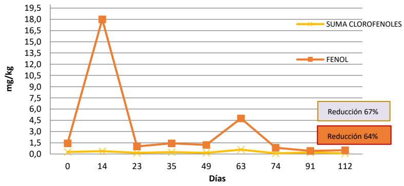
Evolución temporal FENOL Y CLOROFENOLES. Reactor AE6 - con Estiércol
